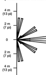
VUE DE CÔTÉ (Détecteur anti-rampement)
